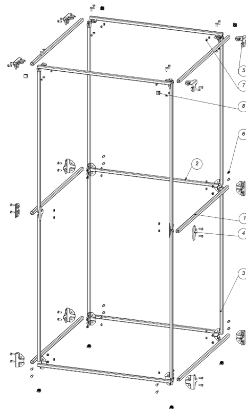
Рисунок 1 – Кабина душевая в разобранном виде Номера позиций проставлены в соответствии с комплектацией (см. Таблицу 2).
